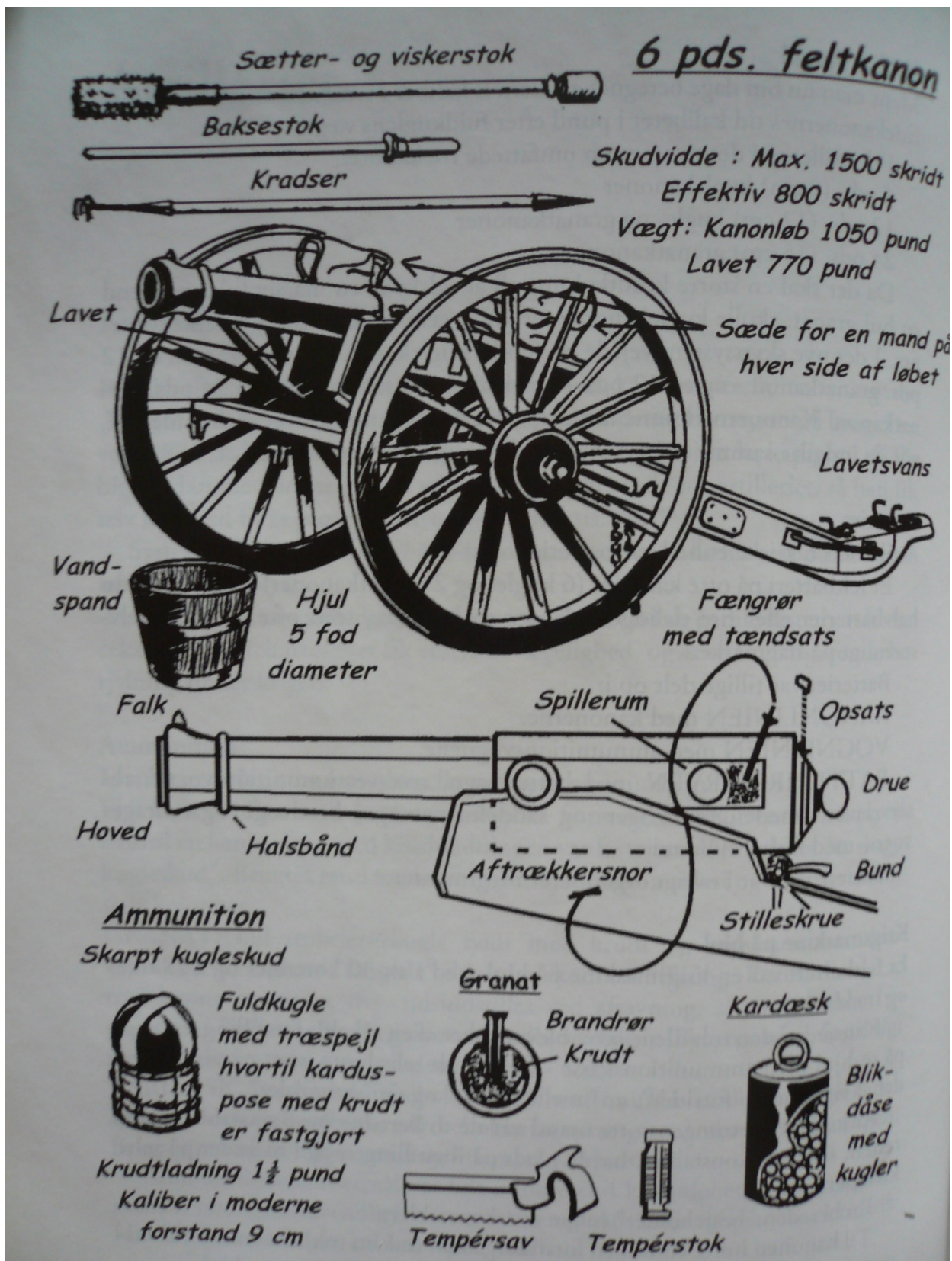
Tegning af 6 pds kuglekanon i lavet af system 1834 med laderedskaber og ammunition
